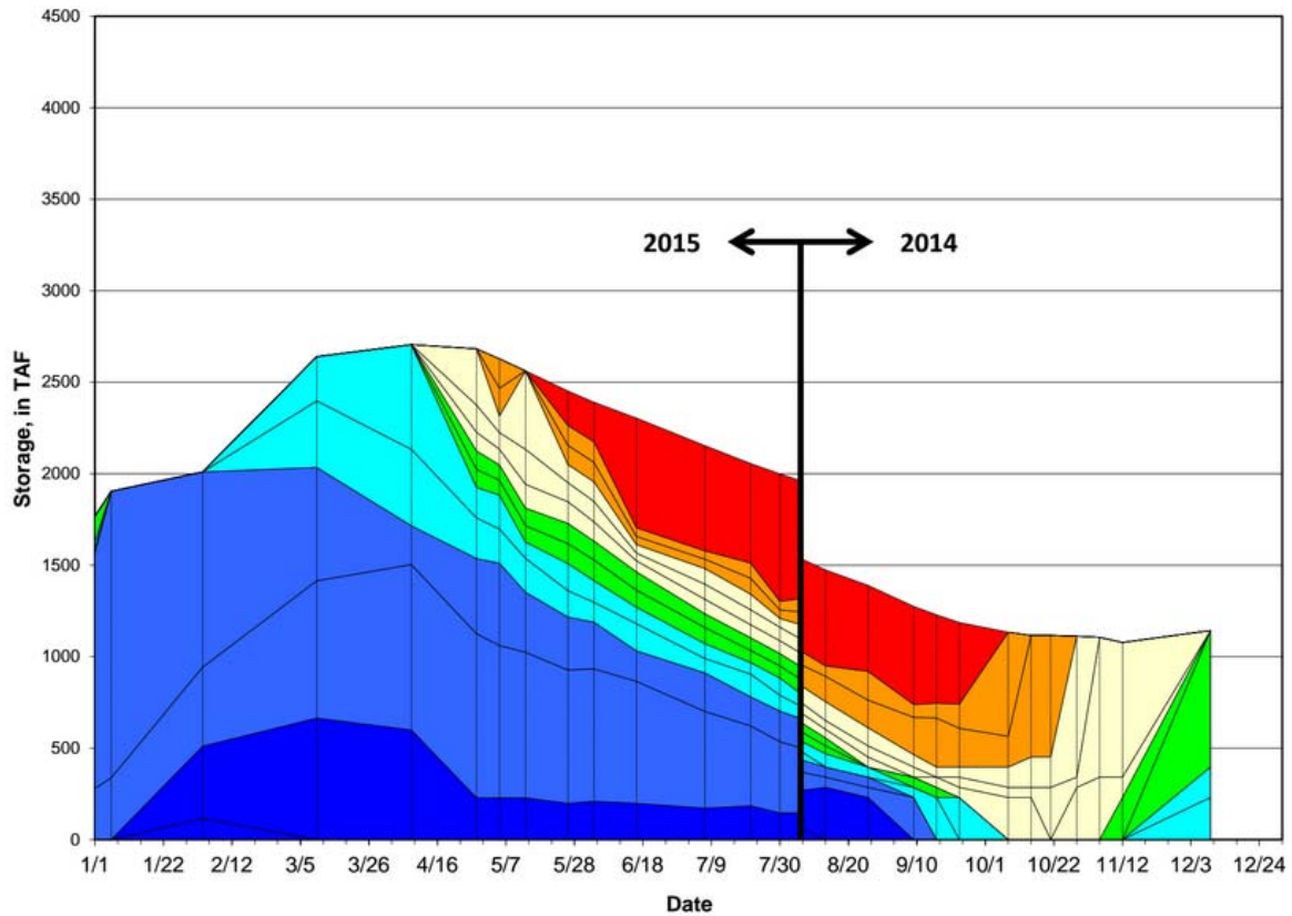
Lake Shasta Isothermobaths (Water Temperature, in ° F)
