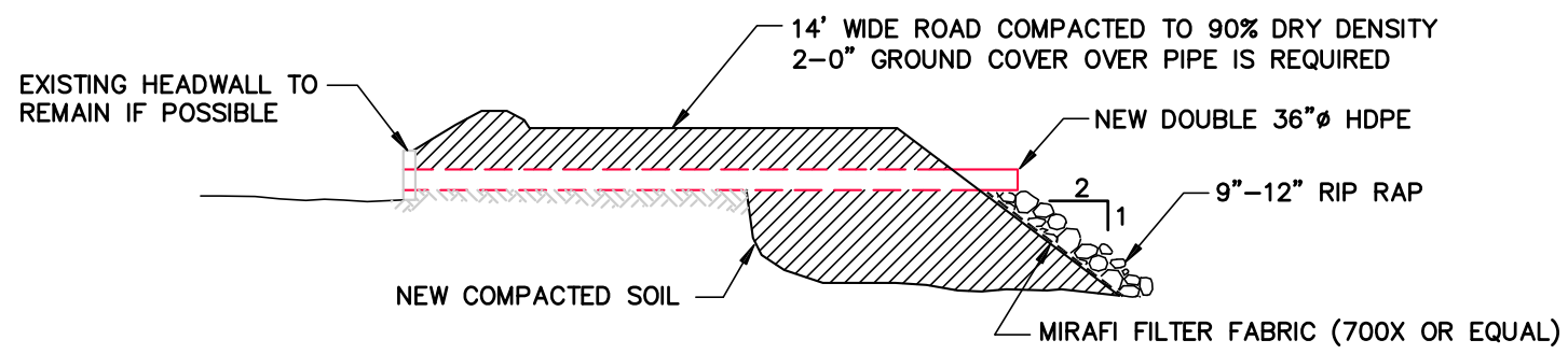
SECTION A-A SCALE: 1" = 10'
