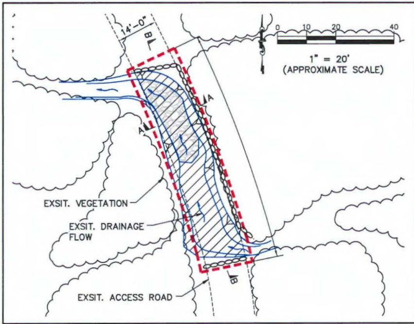
PLAN SCALE: 1' = 20'
