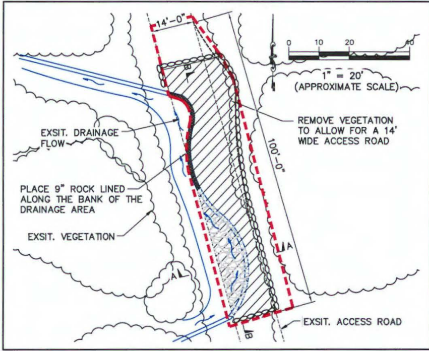
PLAN SCALE: 1" = 20'
